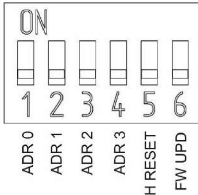
Рисунок 4.6 Назначение DIP-переключателей
