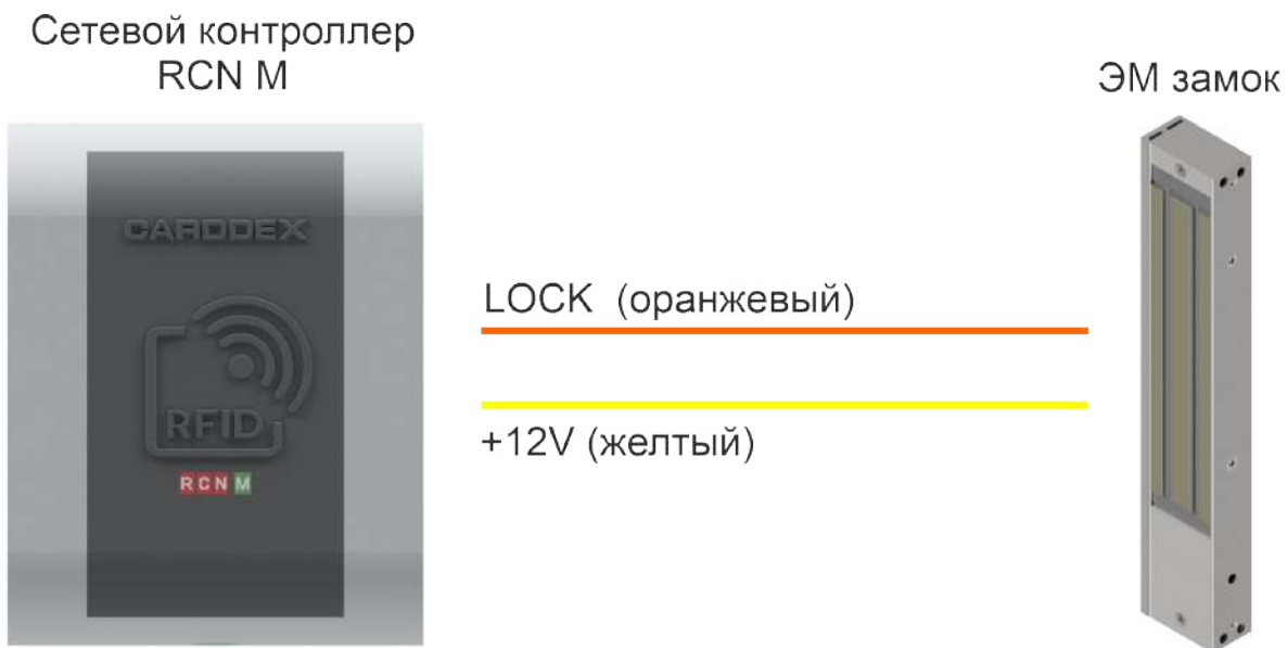
Рисунок 4.4 Подключение запирающего устройства
