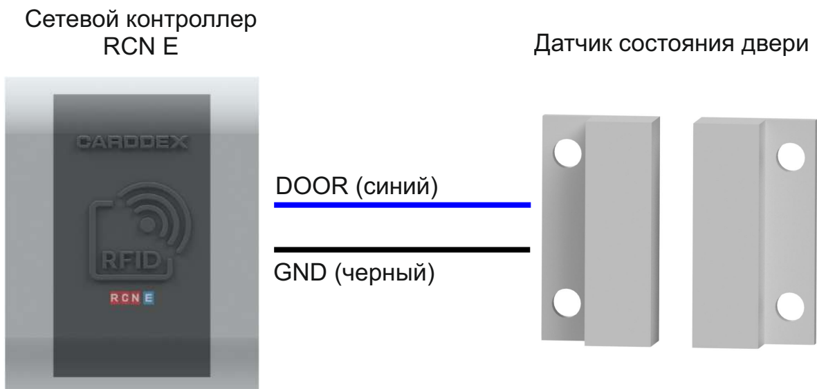
Рисунок 4.3 Подключение датчика состояния двери
